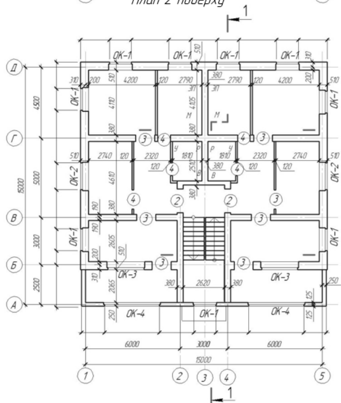
План 2 поверху
