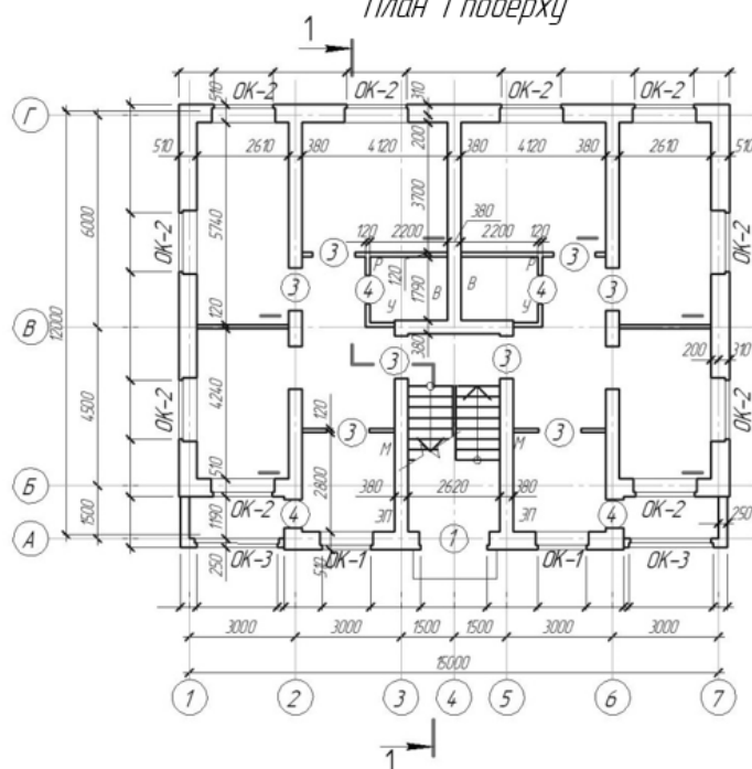
План 1 поверху
