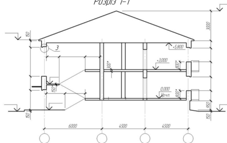
Розріз 1-1
