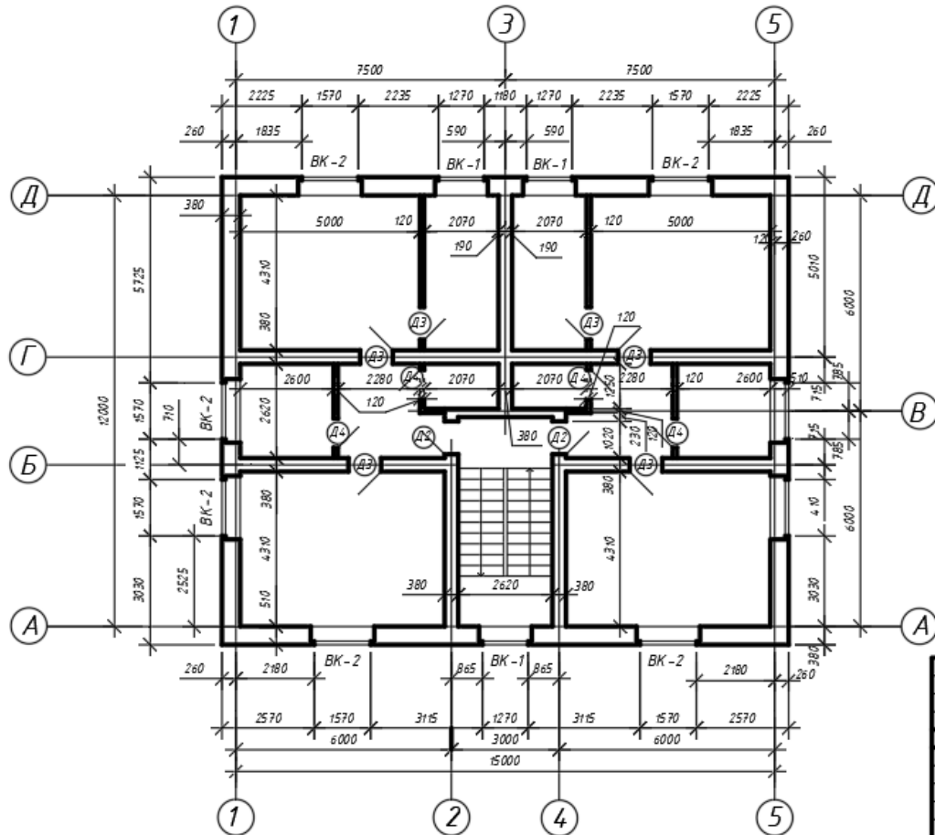
План 2-го поверху
