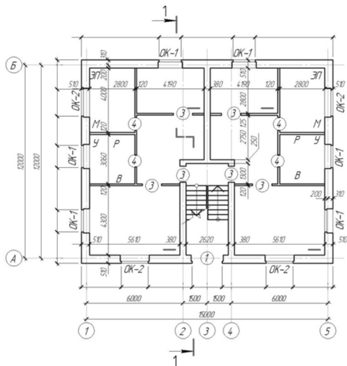
План 1 поверху
