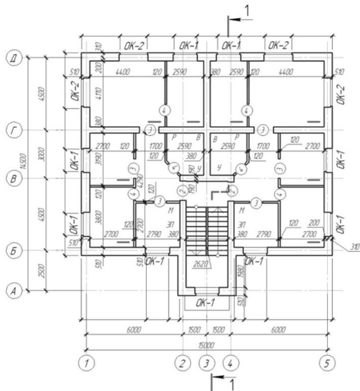
План 2 поверху
