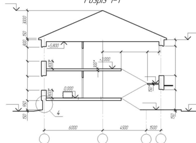
Розріз 1-1
