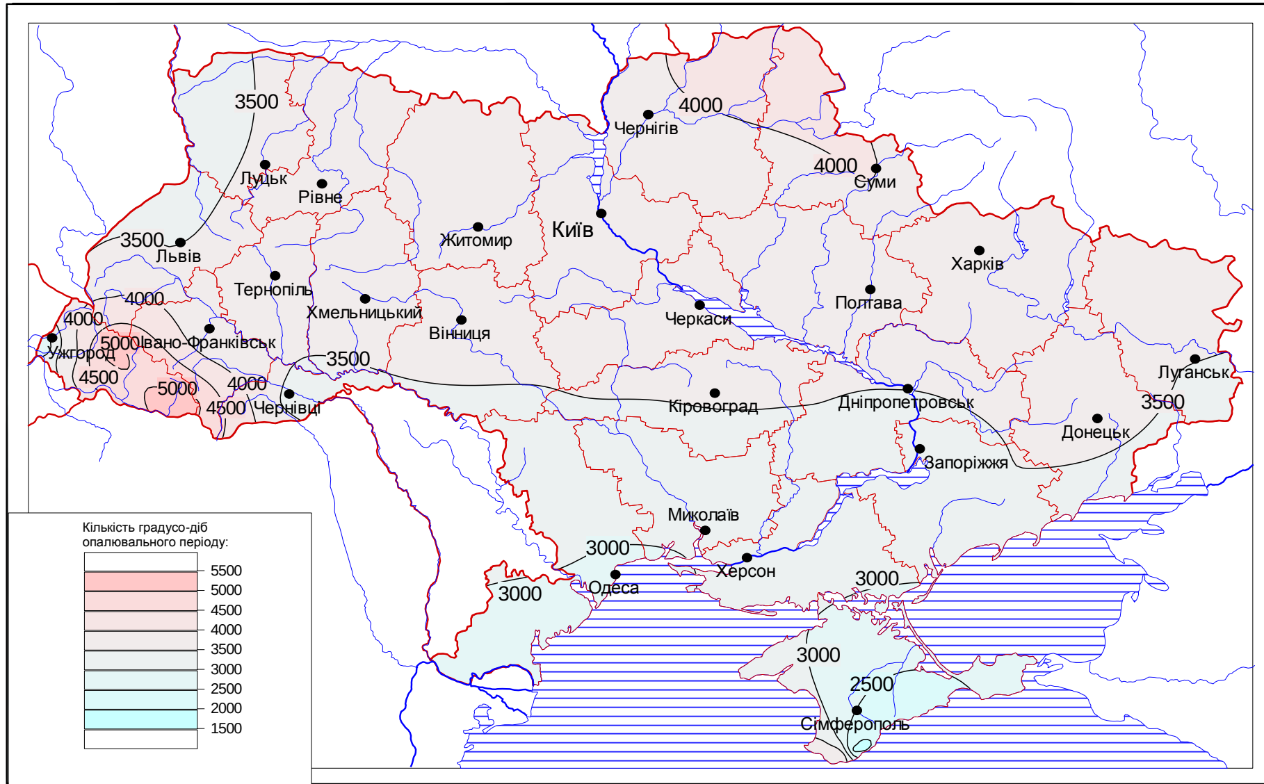
Рисунк 2 – Районування території України за кількістю градусо-днів опалювального періоду
